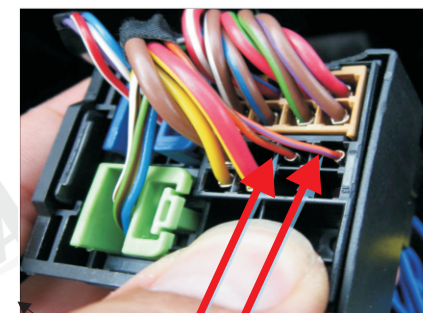
CAN H - oranžovo-fialová CAN- L - oranžovo hnědá
